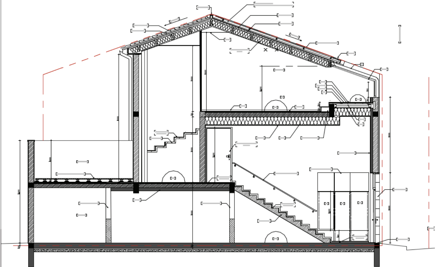
COUPE C02
