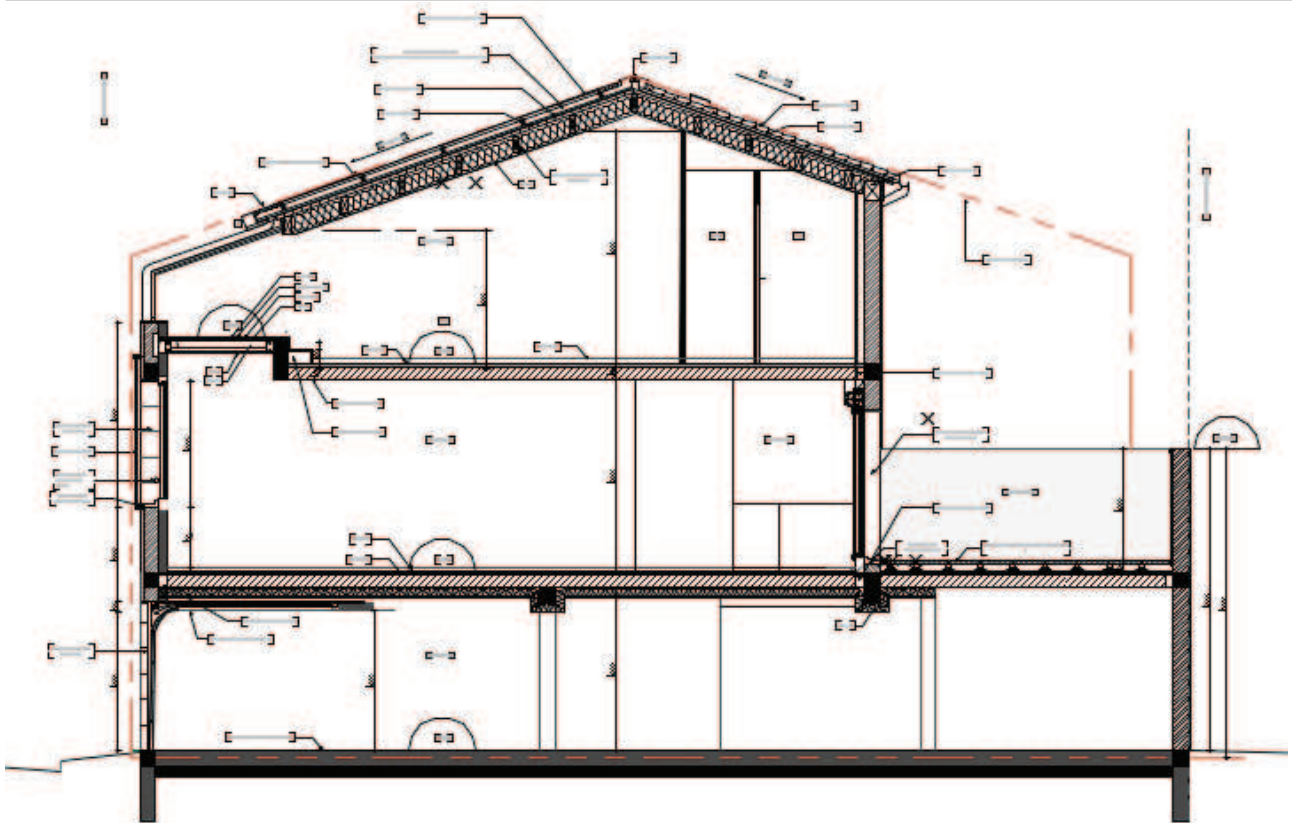
COUPE C03
