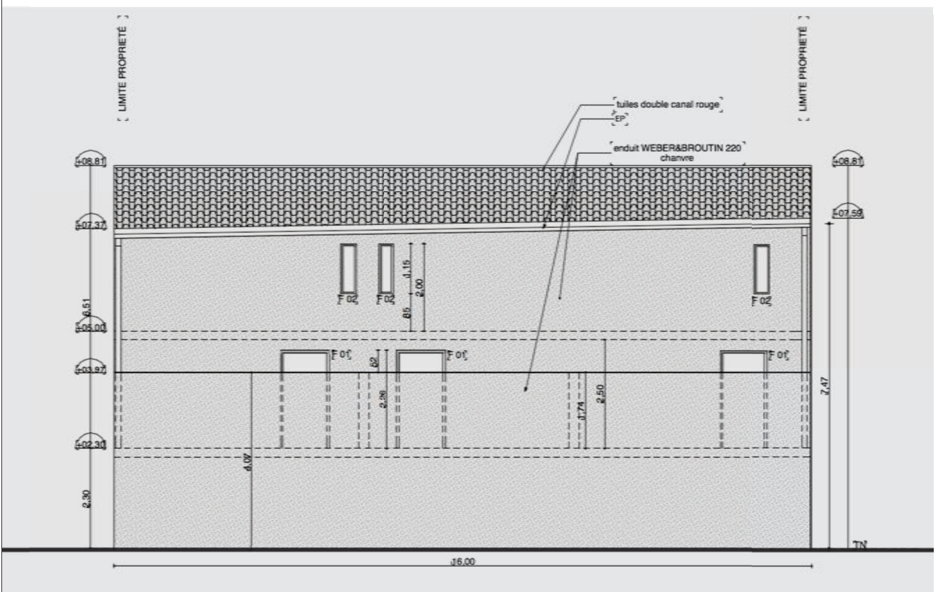
FACADE OUEST
