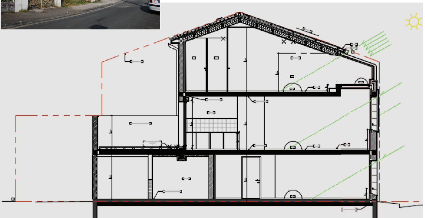
COUPE AA
