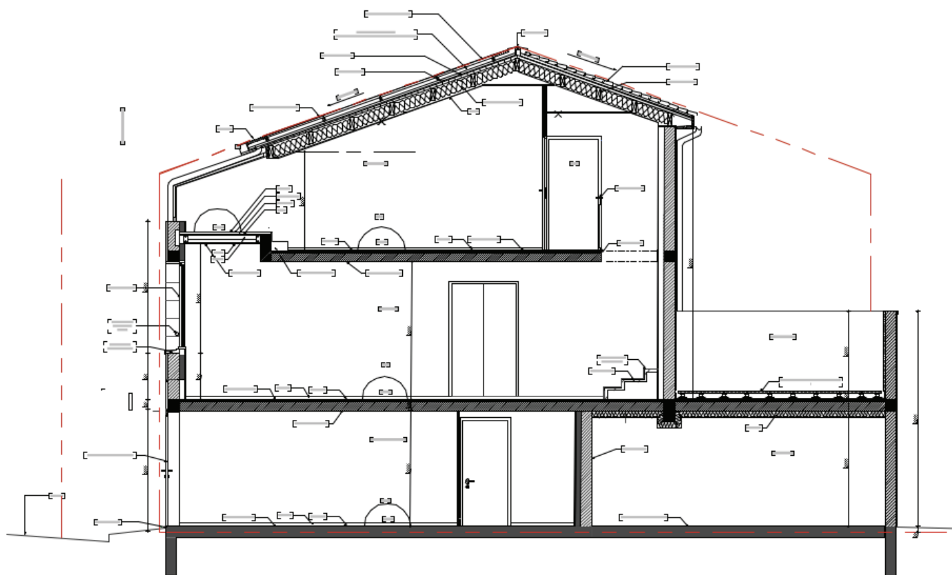
COUPE C04
