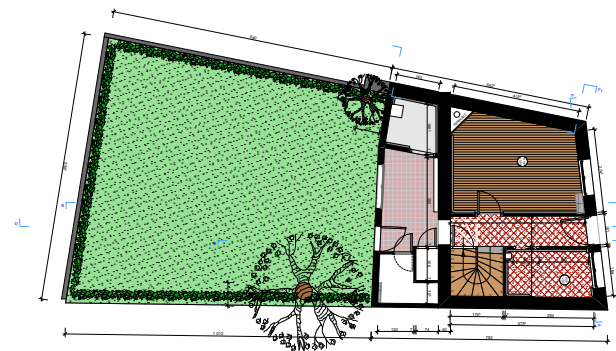
Plan existant RDC 1/200ème
