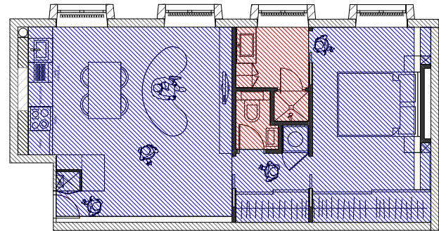
Plan de faux-plafond
