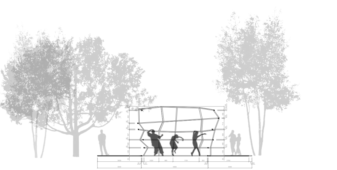
Coupe sur structure centrale 1/75 ime.
