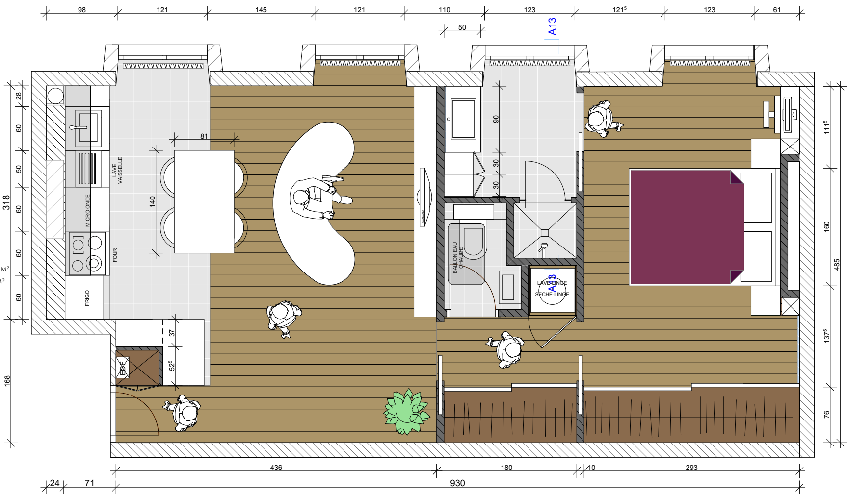
Plan projet 1/50ème
