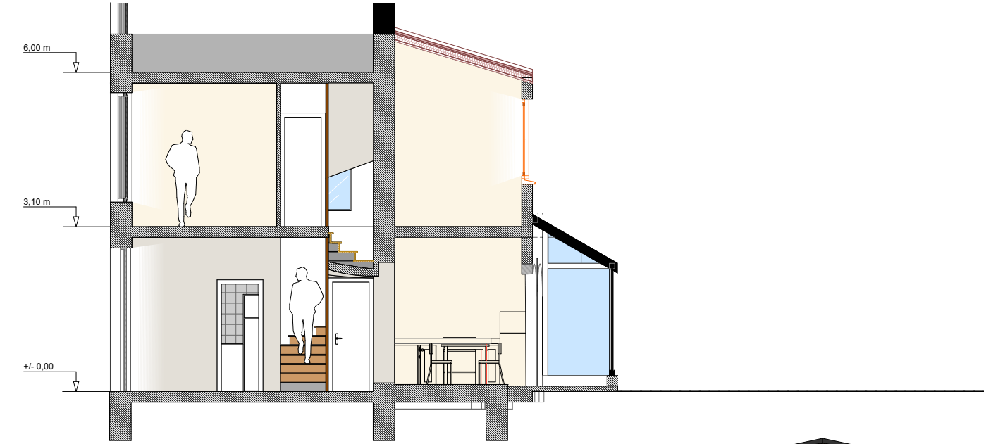
Coupe C-C 1/100ème
