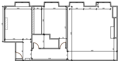
Plan existant 1/200ème
