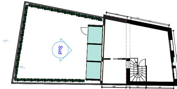
Plan projet R+1 1/200ème
