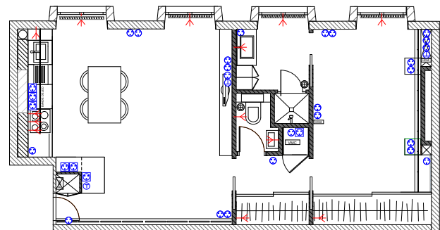
Plan d'électricité
