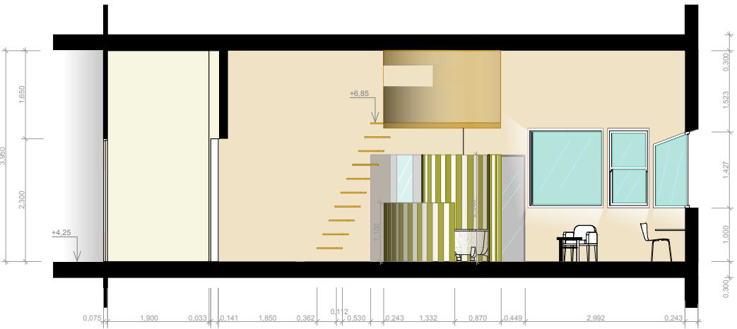
COUPE A-A 1/100 EME
