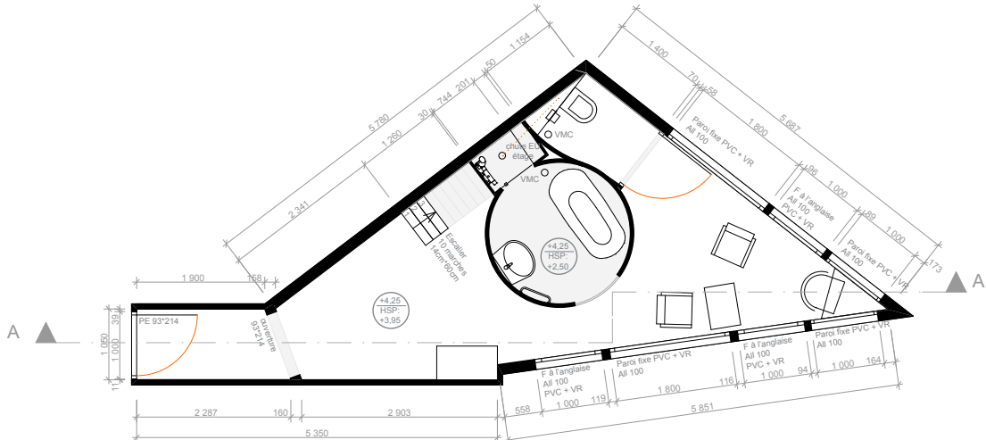
PLAN SUR 1ER NIVEAU 1/100 EME
